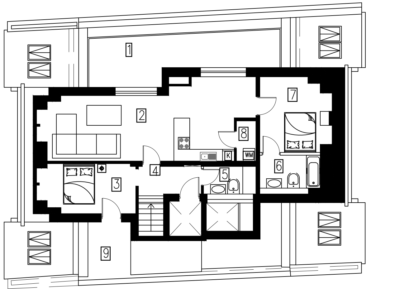
TOP 10 Dachgeschoß
